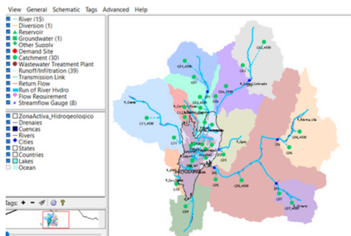
Fuente: SEI. Vista esquemática del modelo hidrológico WEAP ( Water Evaluation and Planning System ) de la cuenca del Salar de Pastos Grandes.
